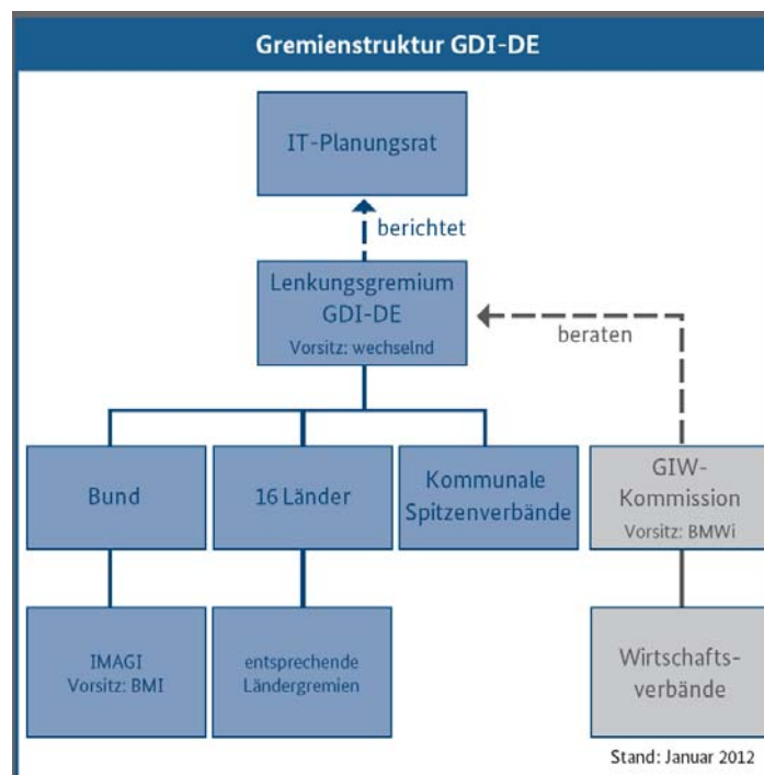
Abb. 2: Gremienstruktur GDI-DE
